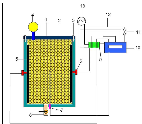
شكل (3): مخطط لاستخلاص مضادات الأكسدة بالتسخين الأومي (Al-Hilphy et al. , 2020) (1: غطاء الاسطوانة، 2: عينة، 3: برغي، 4: مقياس الضغط، 5: قطب كهربائي، 6: برغي، 7: مزدوج حراري، 8: صمام، 9: موصل، 10: مقياس درجة الحرارة الرقمي، 11: مفتاح تشغيل، 12: توصيل الأسلاك، 13: امدادات الطاقة.
