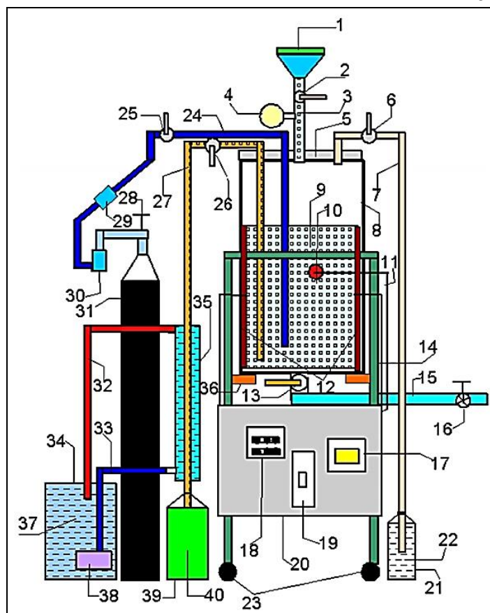
شكل (6): جهاز استخلاص الأحماض الأمينية بالماء تحت الحرج والتسخين الأومي معاً (Kadem et al. , 2023)
